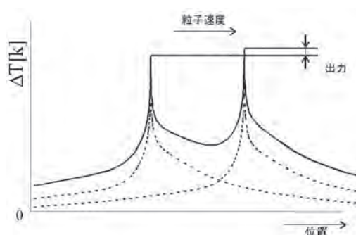
空気粒子が熱線から熱を奪う。進行方向により 2 本の熱線に温度差が生じる。 この差が粒子速度のレベルとして計測される。
