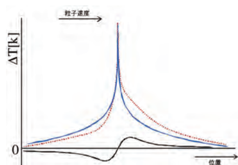
熱線の周囲の温度変化 青線 - 粒子速度無し 赤線 - 粒子速度有り
