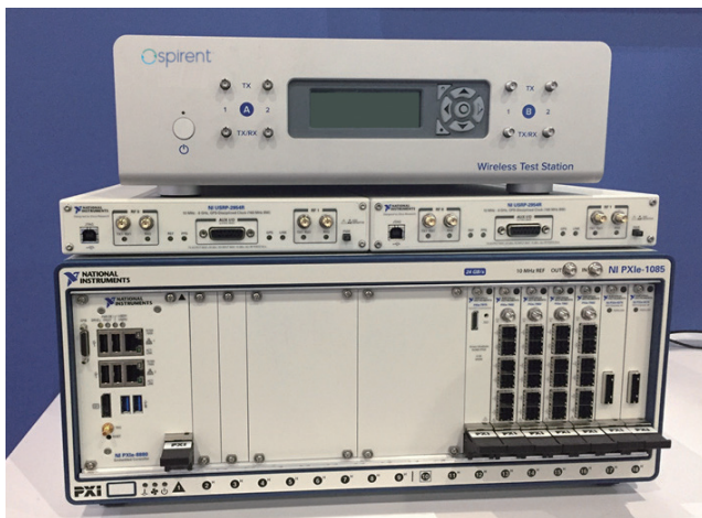
【5G NSAシミュレーションシステム】 SR9860 5G gNBシミュレータ + WTS122 LTE eNBシミュレータ
