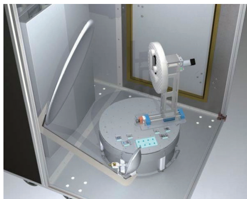
5Gオプション実装イメージ
