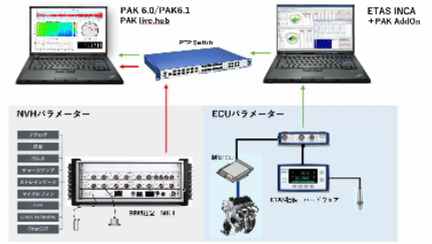
NVHとECU内部データの 統合計測システム 概要
