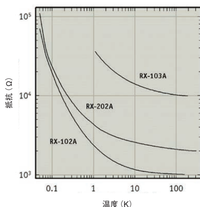
RX シリーズ抗温度計の抵抗温度特性と感度
